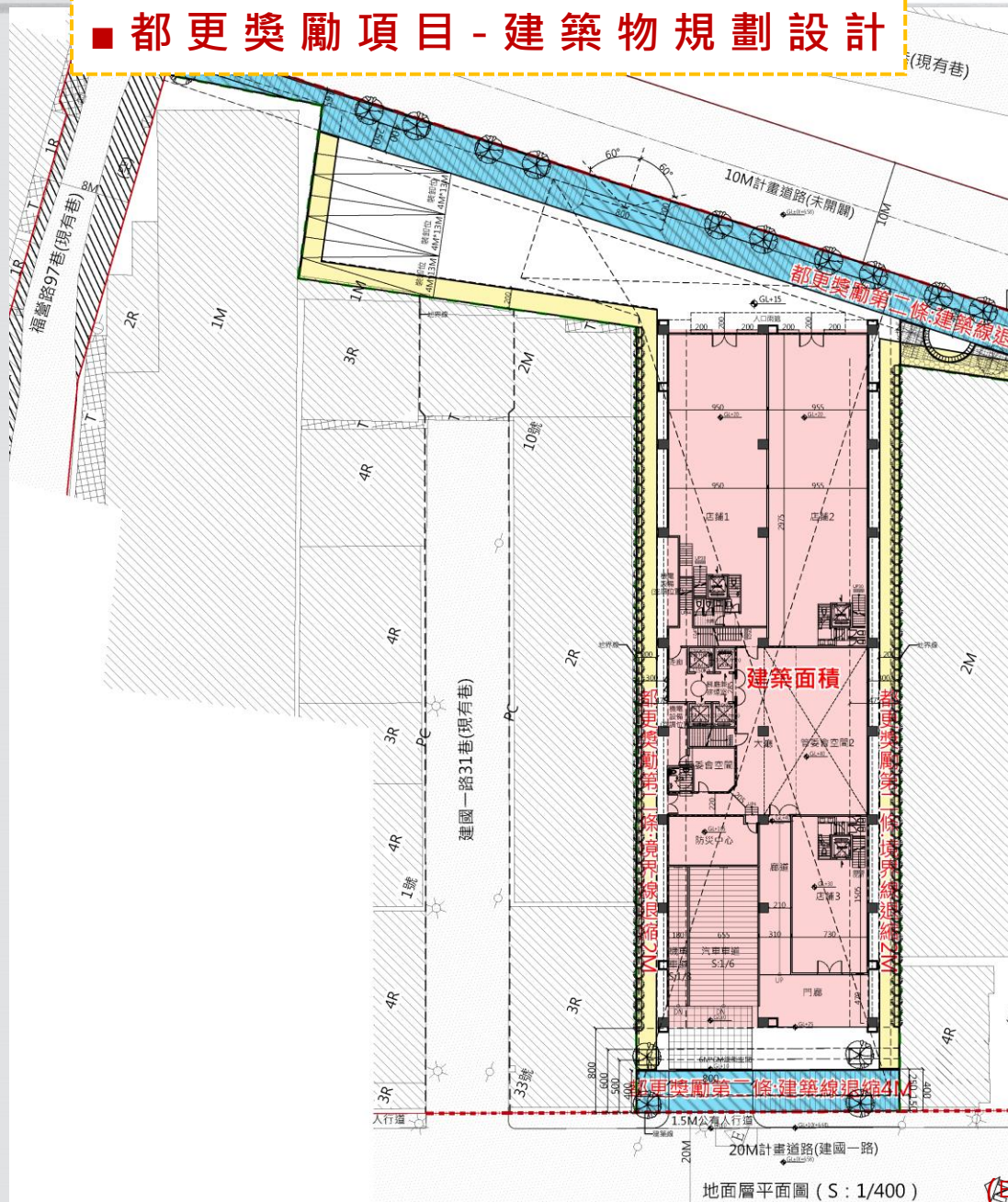
地面層平面圖 (S: 1/400)
