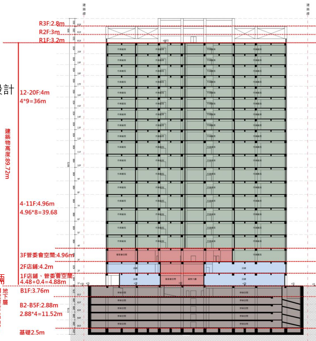
長向剖面圖
